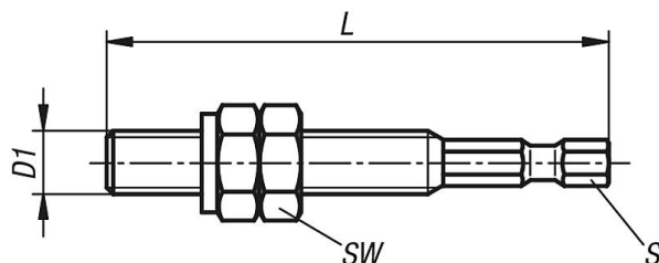
Outil de montage manuel
