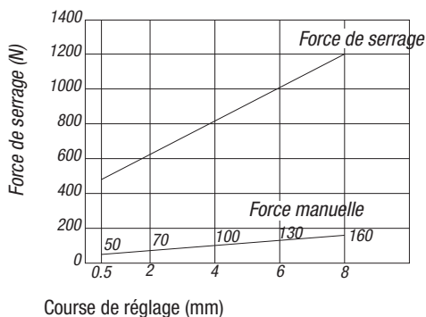
Bride pivotante 04366-...4540
