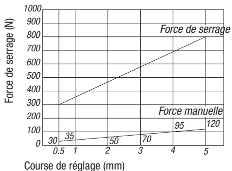
Bride pivotante 04366-...3232
