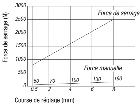
Vérin à tirer 04400-4050...
