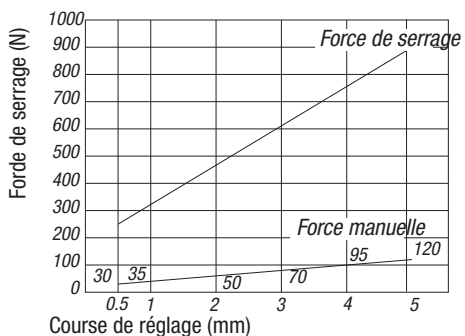
Vérin à tirer 04400-3240...
