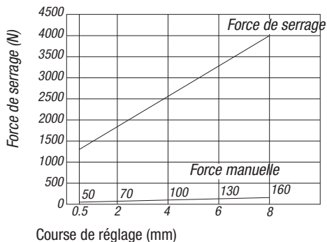
Crampon plaqueur 04565-0800 Crampon plaqueur 04565-0801
